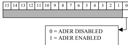
Fig. 6.13: Enable ADER Register
